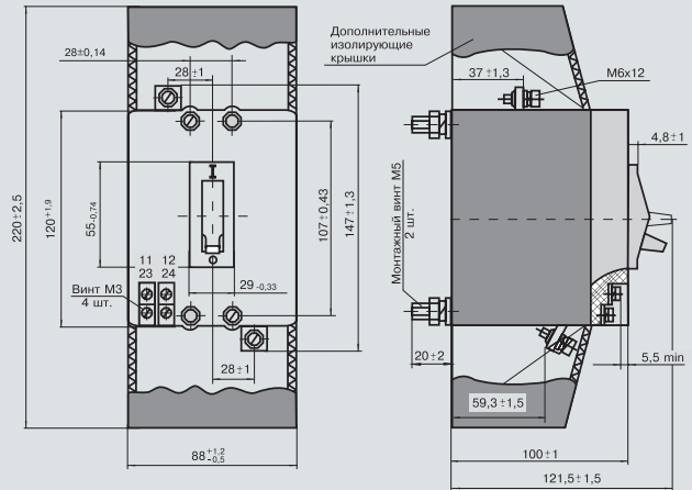
однополюсный выключатель BA21 в трехполюсном габарите
